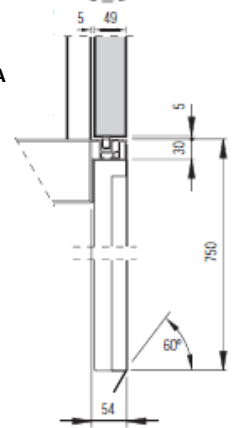
DETAY A
